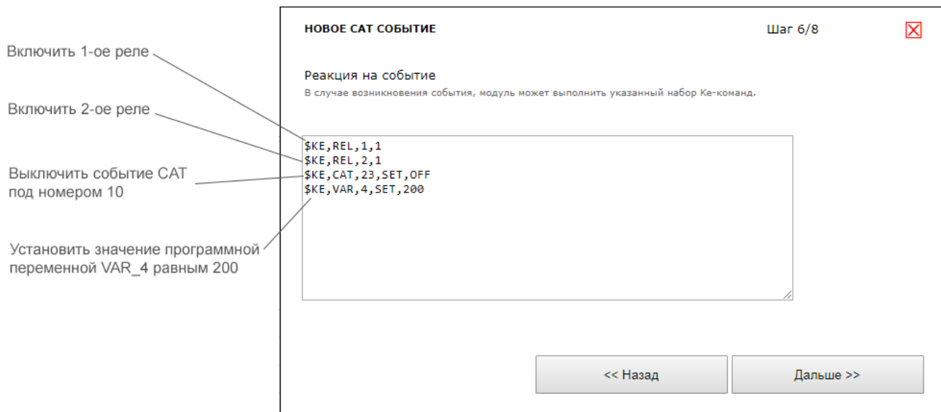
Рис. Система САТ. Шаг 6 – задание реакции при срабатывании события в виде списка Ке-команд.
